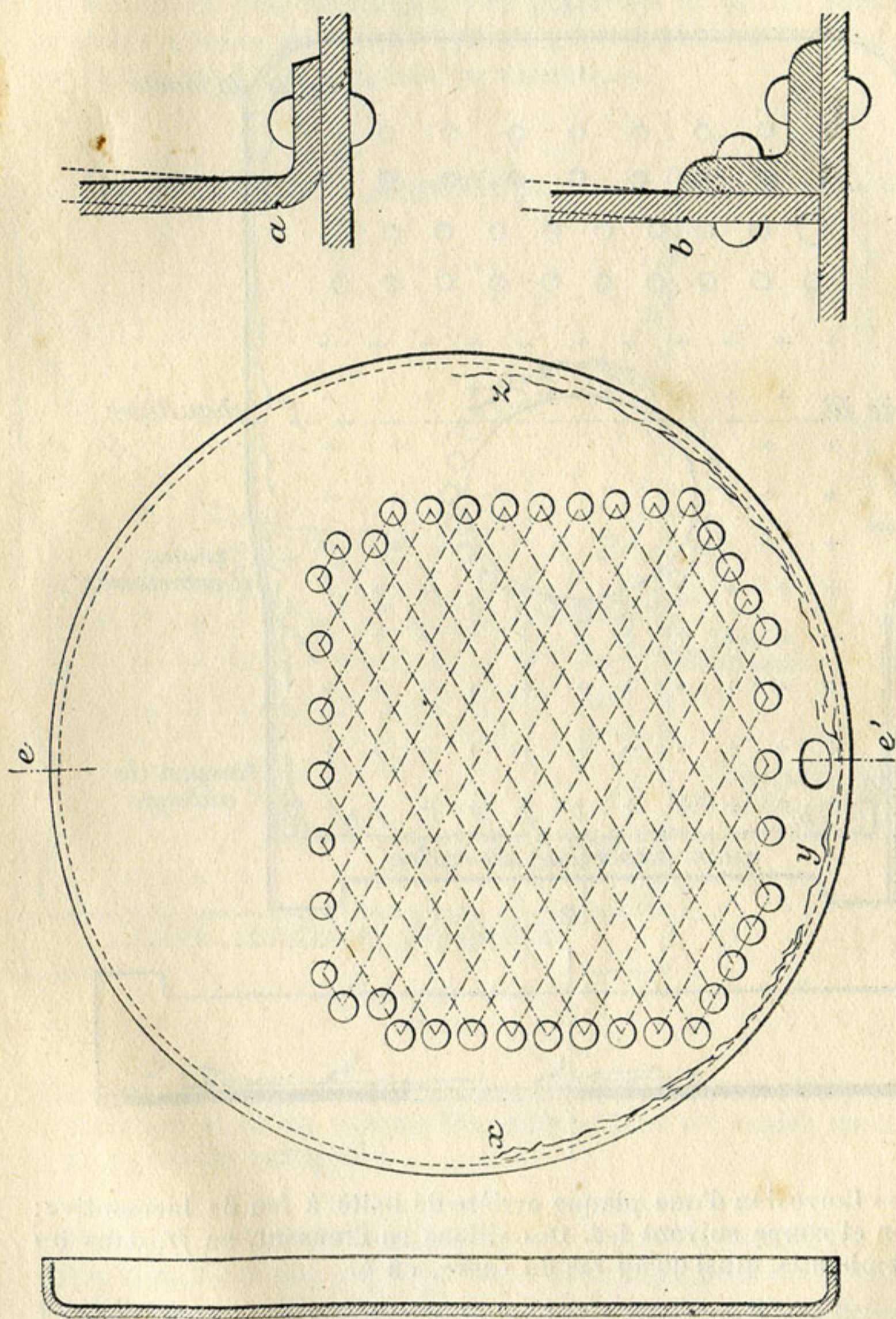
Fig. 322. — Corrosion d'une plaque tubulaire de boîte à fumée de locomotive. Le bord embouti de la plaque, en contact avec l'eau, se ronge en a suivant la demi-circconférence inférieure xy . Les plaques fixées par une cornière se rongent en b .
