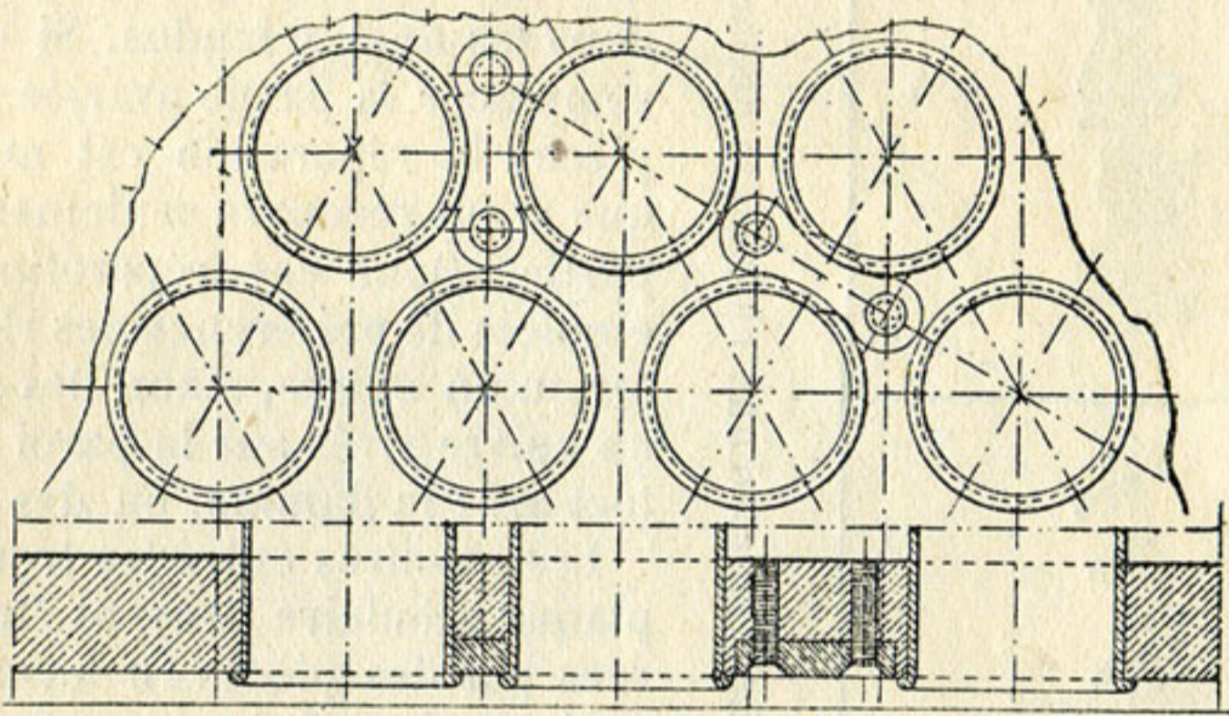
Fig. 320. — Réparation des cassures des plaques tubulaires.
