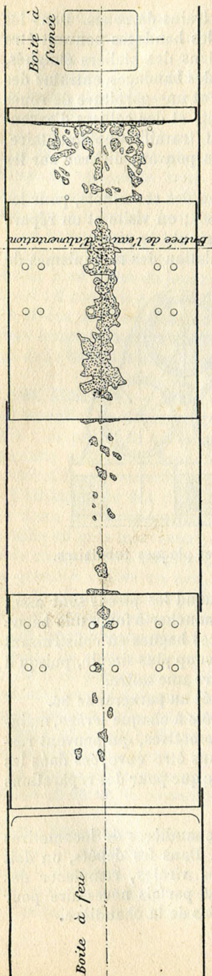
Fig. 321. — Corrosions intérieures à la partie inférieure d'une chaudière de locomotive; vue en plan.
